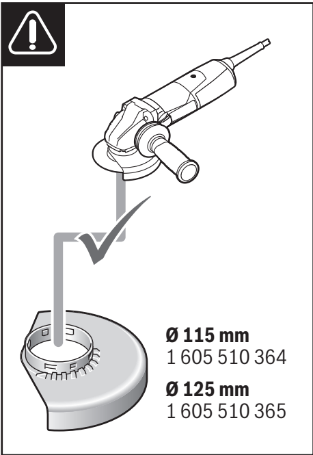
GDE 115/125 FC-T 1 600 A00 3DK
